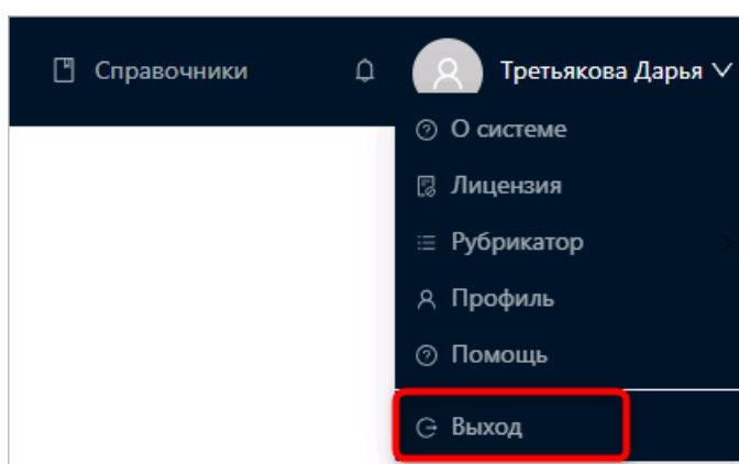
Рисунок 16 – Завершение работы
