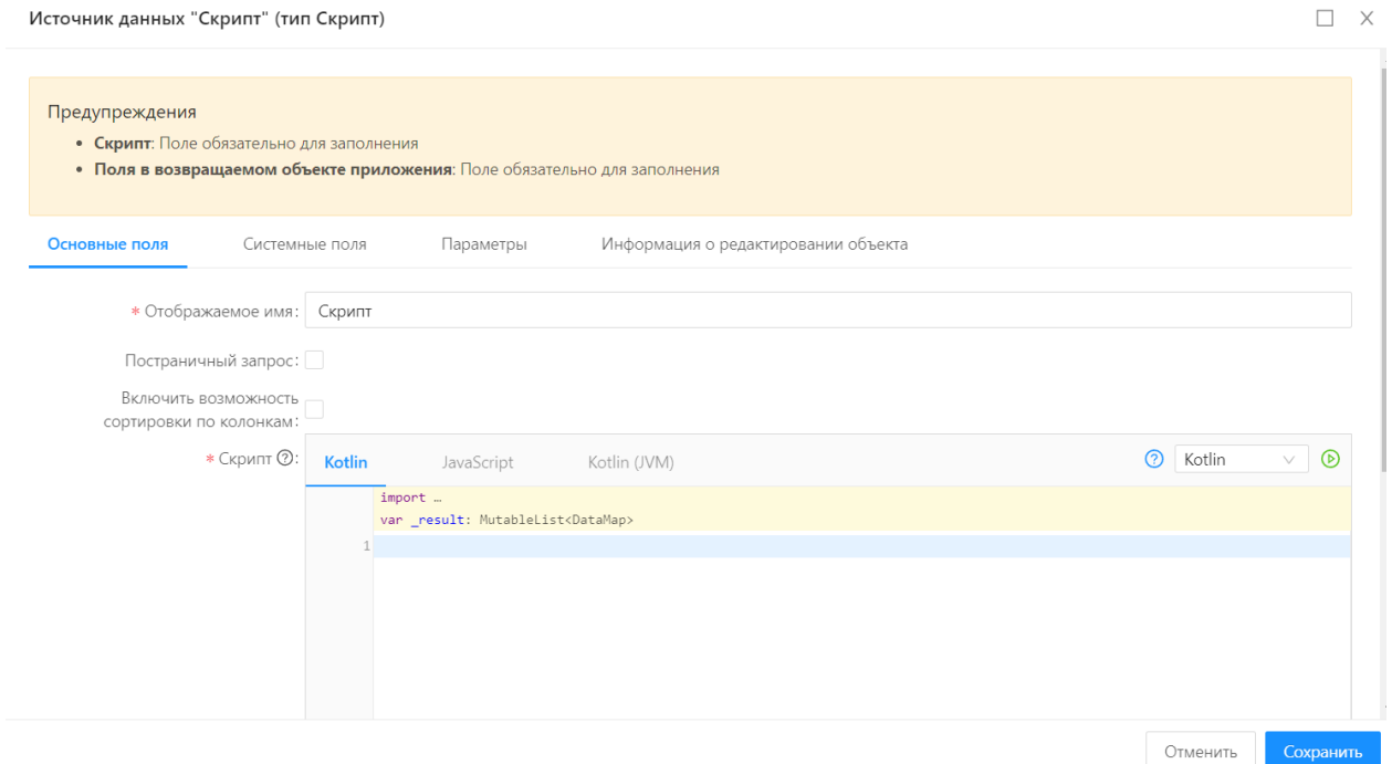
Рисунок 14.55. Настройка источника данных «Скрипт»
