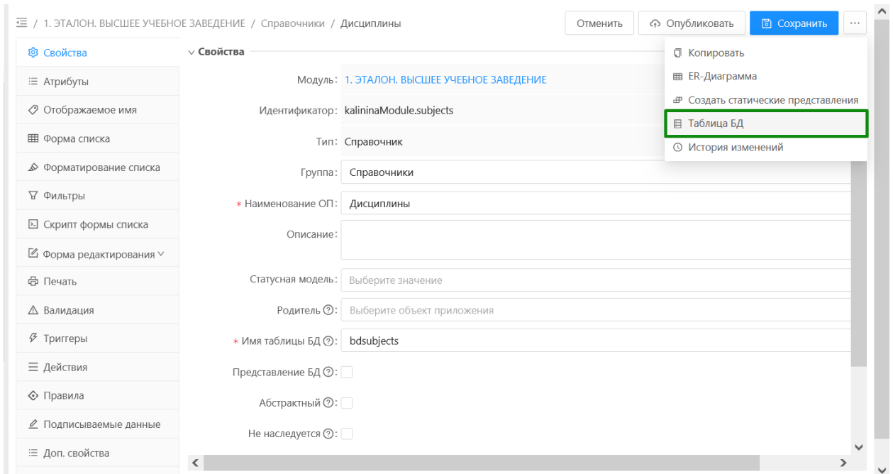
Рисунок 8.1 – Действие «Таблица БД» в конфигурации объекта приложения
