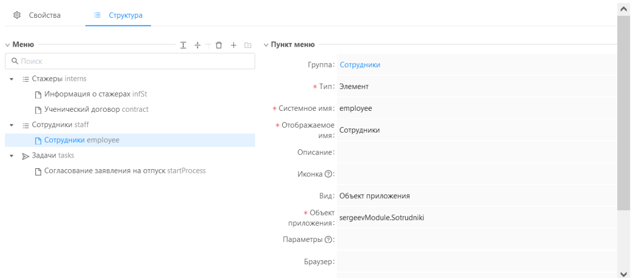
Рисунок 3.11 – Вкладка «Структура» рубрикатора»
