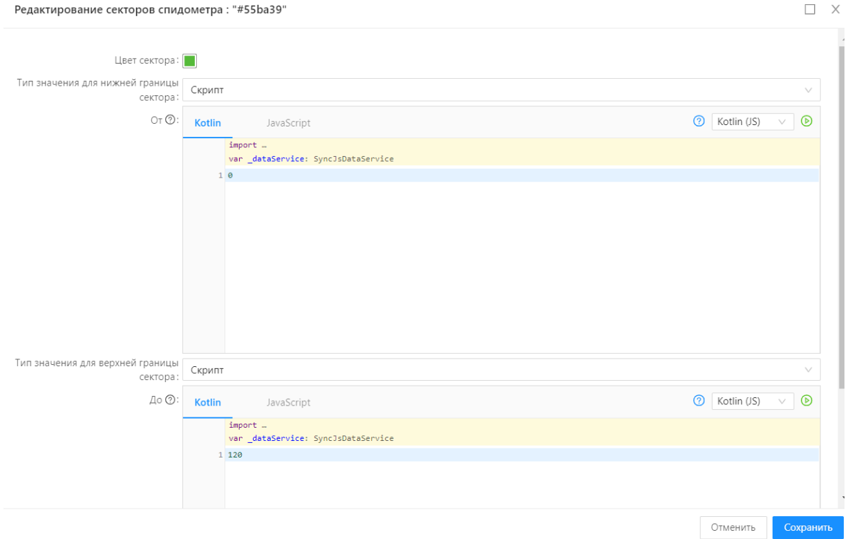
Рисунок 14.180. Настройка секторов виджета «Спидометр»
