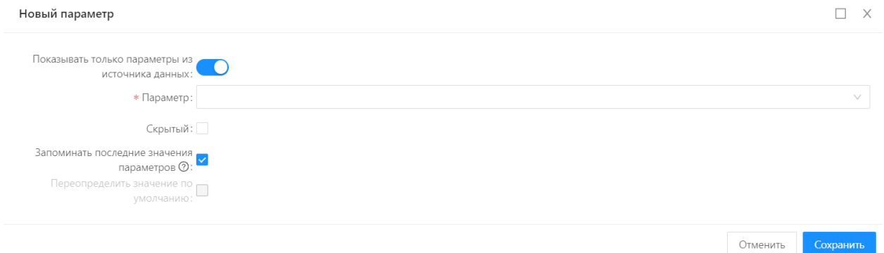
Рисунок 14.105. Форма редактирования/создания локального параметра виджета
