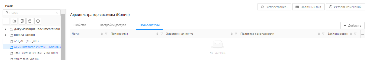
Рисунок 5.5 – Вкладка «Пользователи»
