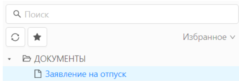
Рисунок 11.7 – Просмотр избранного
