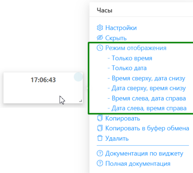
Рисунок 14.306. Доступные режимы отображение виджета «Часы»
