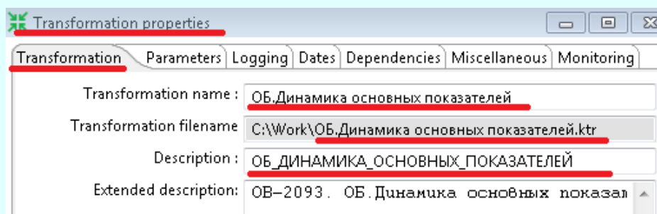
Рисунок 25 – Закладка «Transformation»
