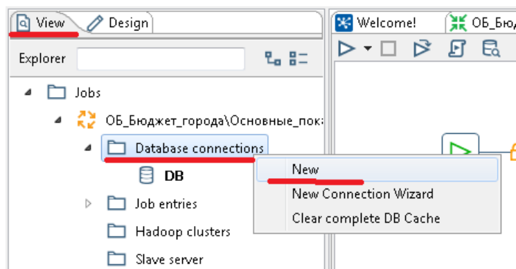
Рисунок 19 – Закладка «View»
