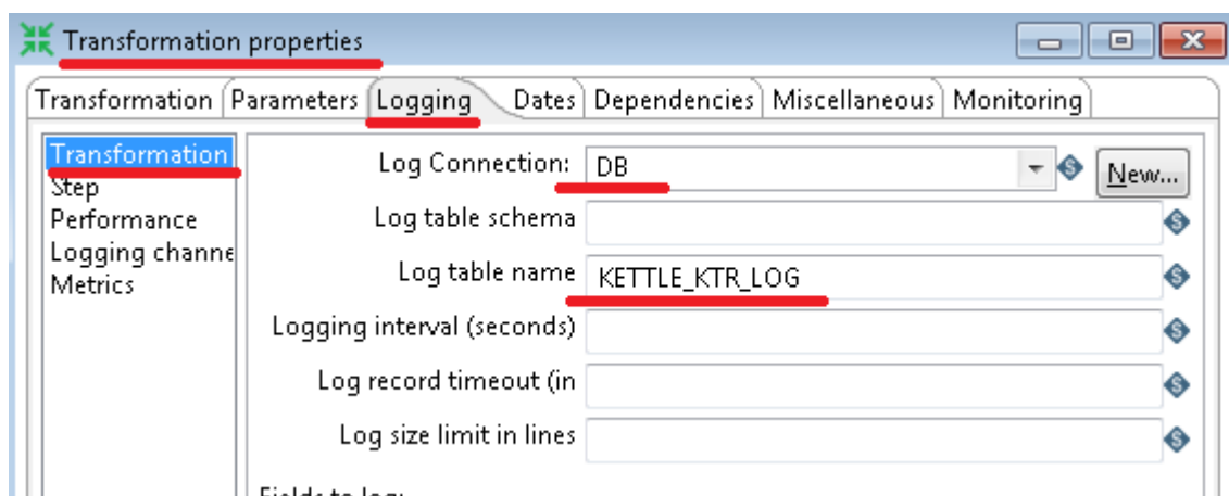
Рисунок 26 – Закладка «Logging»
