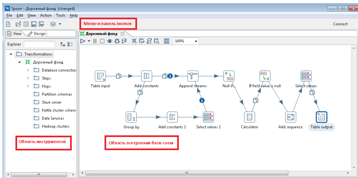
Рисунок 18 – Графический интерфейс
