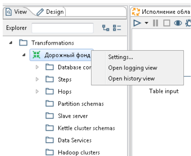
Рисунок 24 – Закладка «View»
