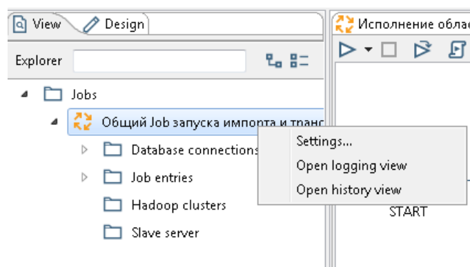
Рисунок 27 – Закладка «View»
