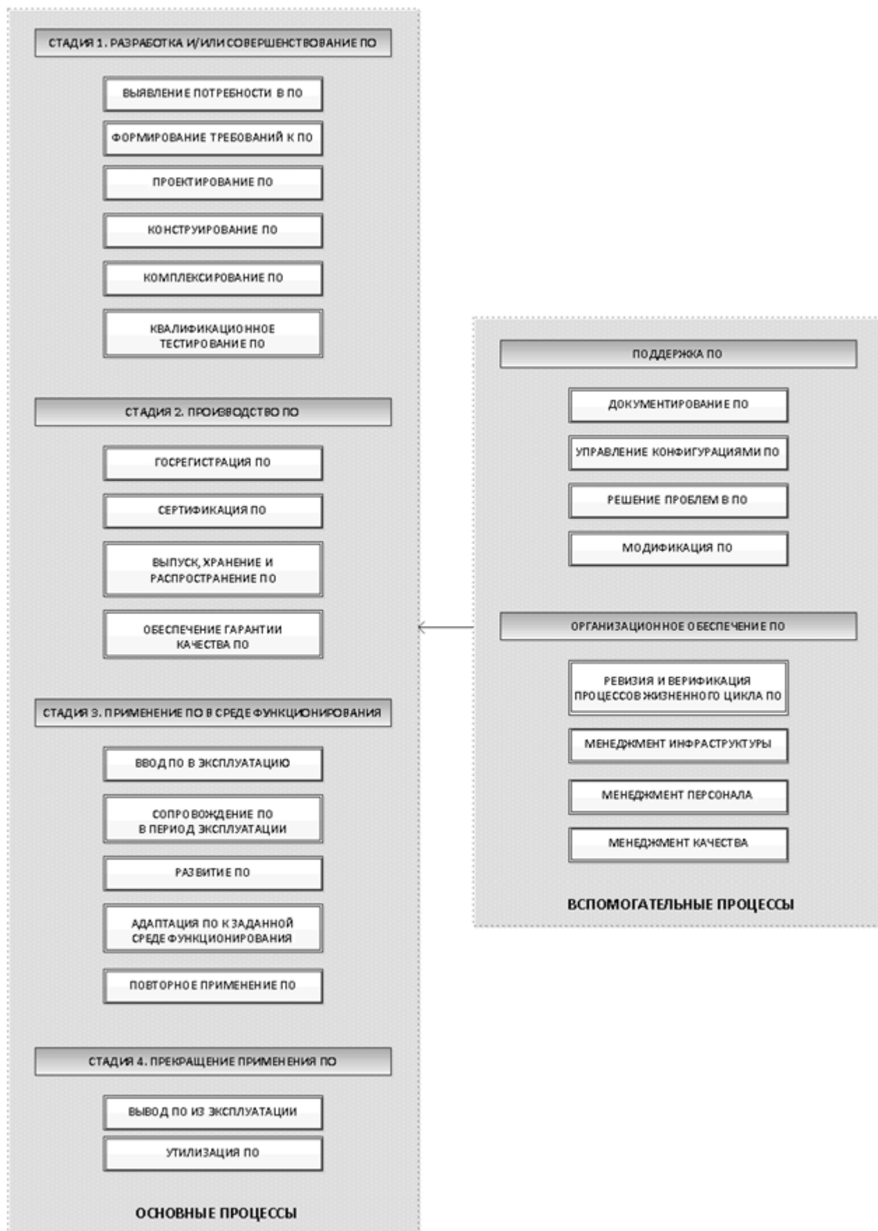
Рисунок 1. Модель жизненного цикла программы для ЭВМ «Комплекс программ «БФТ.Платформа»»
