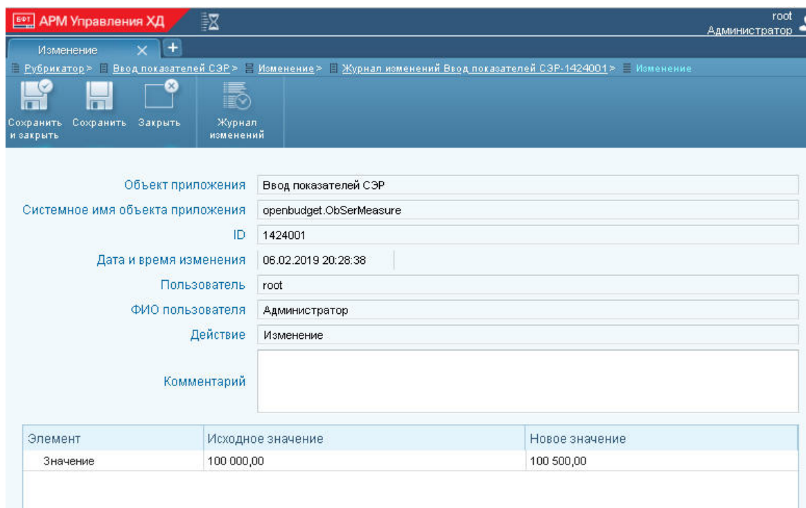
Рисунок 8 – Изменение записи «Журнала изменений»
