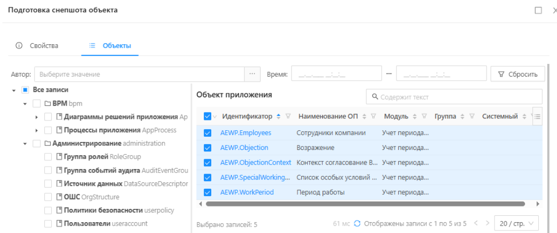
Рисунок 8.138 – Форма подготовки снимка объекта на вкладке «Объекты»
