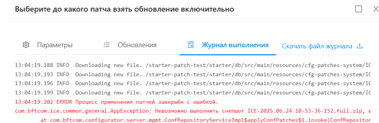
Рисунок 8.162 – Вкладка «Журнал выполнения» в окне выбора патча для обновления
