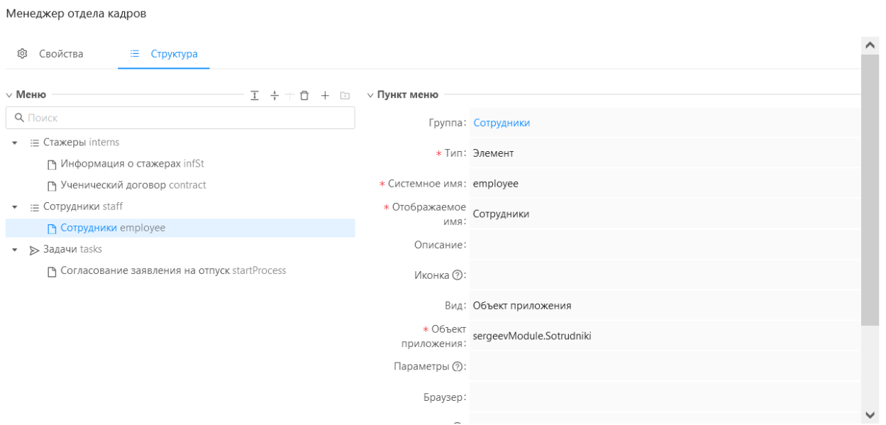
Рисунок 3.11 – Вкладка «Структура» рубрикатора»
