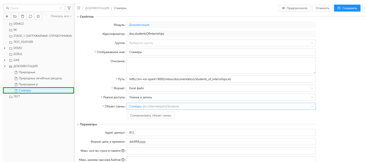
Рисунок 20.3 – Созданная запись в справочнике «Источники данных»
