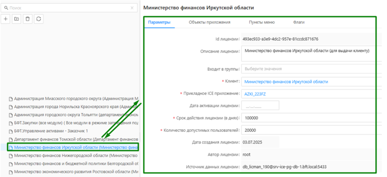
Рисунок 13.6 – Форма просмотра Лицензии
