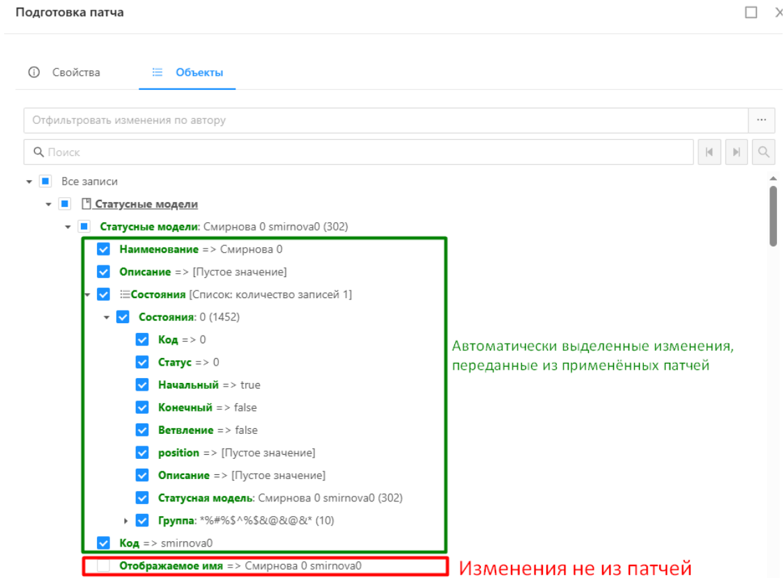
Рисунок 8.165 – Выделенные изменения из применённых патчей в окне подготовки патча
