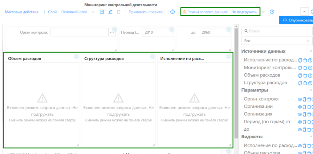
Рисунок 11.297. Пример использования режима запроса данных «Не подгружать»
