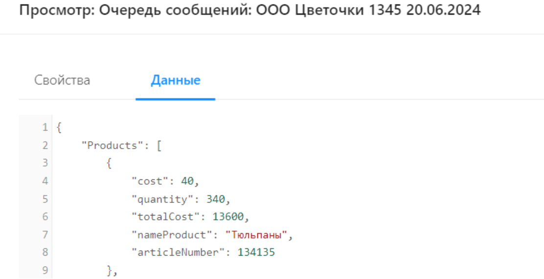
Рисунок 14.38. Форма просмотра сообщения в справочнике «Очередь сообщений» на вкладке «Данные»
