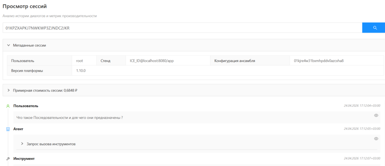
Рисунок 29.16 – История диалога с ИИ-ассистентом
