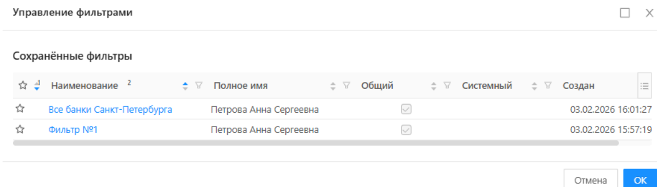
Рисунок 4.68 – Сохраненные фильтры
