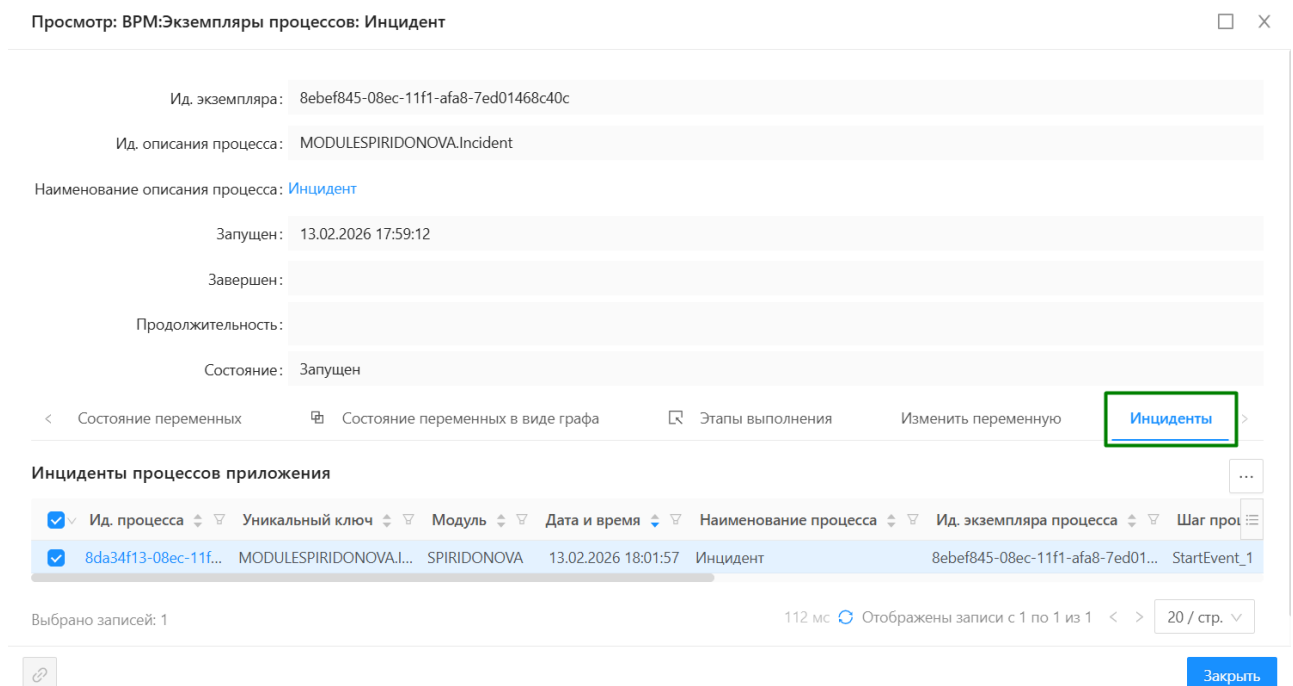
Рисунок 10.100 – Вкладка «Инциденты»
