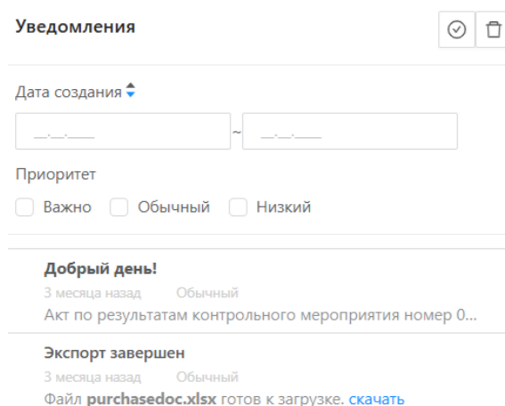
Рисунок 2.3 – Лента уведомлений
