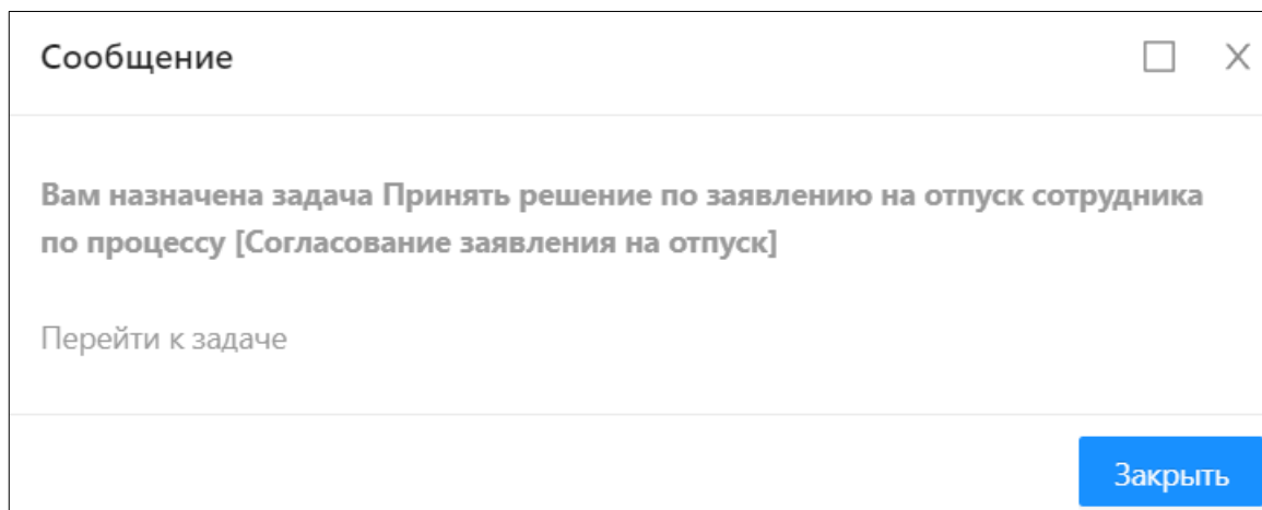
Рисунок 5.8 – Просмотр сообщения
