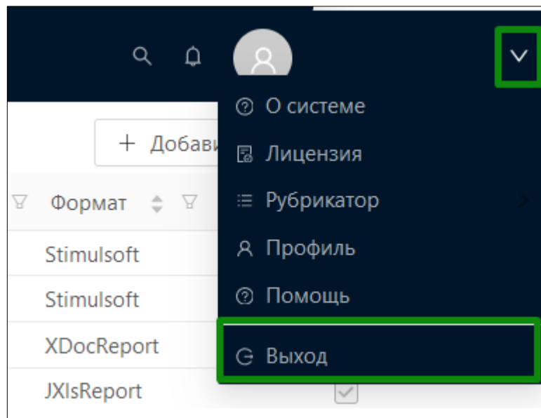
Рисунок 24.1 – Рубрикатор системы
