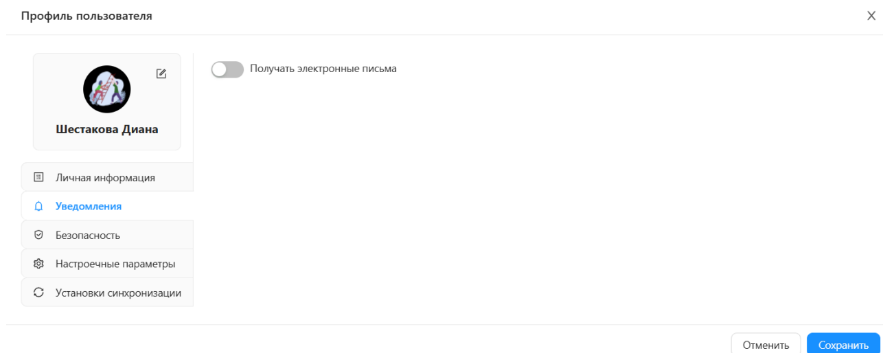
Рисунок 2.48 – Вкладка «Уведомления»
