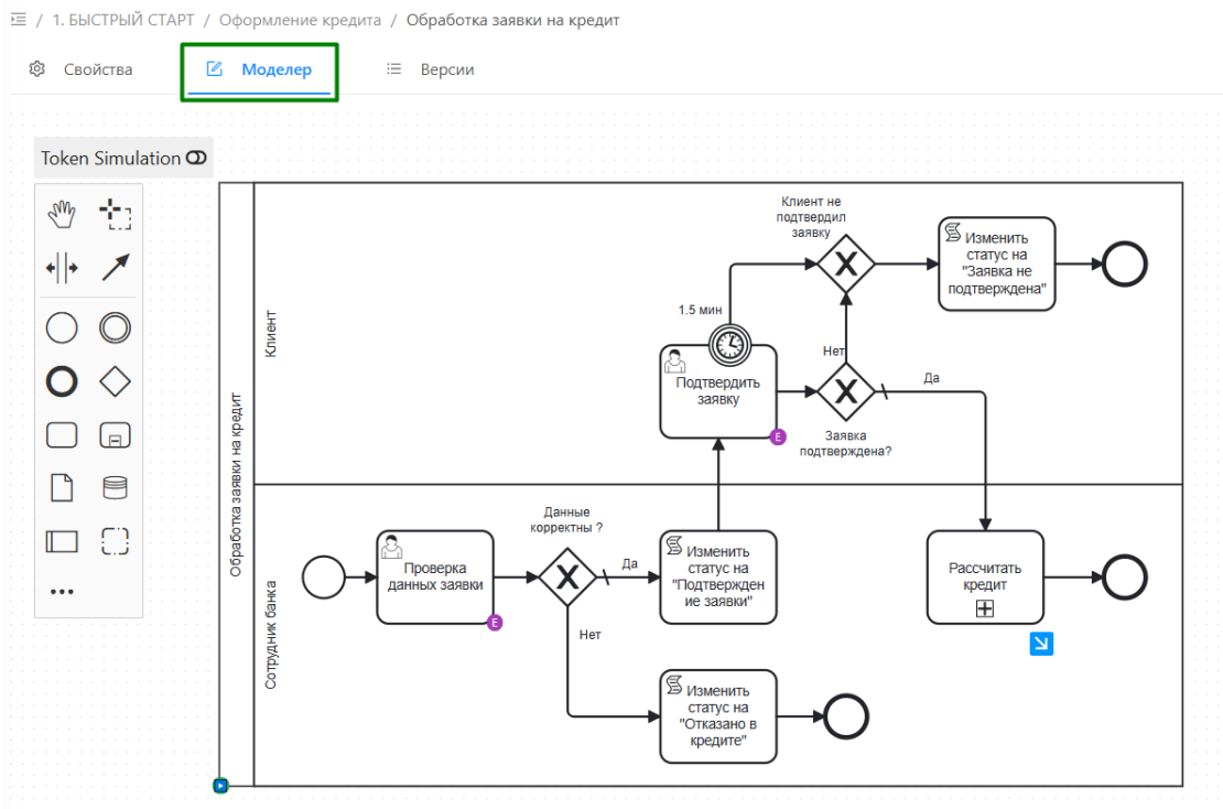
Рисунок 10.21 – Вкладка «Моделер»
