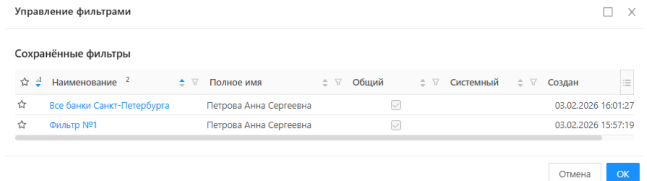
Рисунок 4.72 – Сохраненные фильтры
