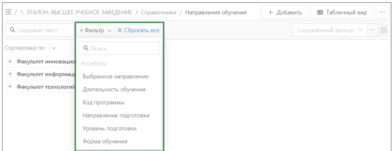
Рисунок 4.37 – Фильтры справочника
