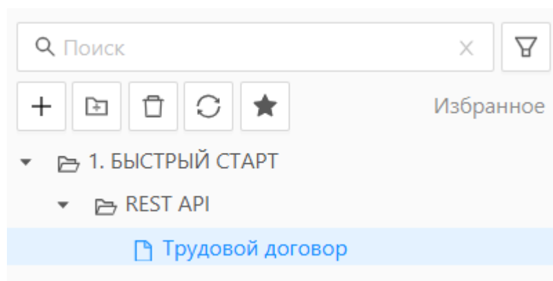
Рисунок 2.33 – Просмотр избранного
