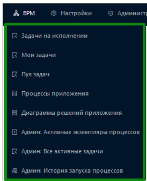
Рисунок 10.1 – Разделы BPM
