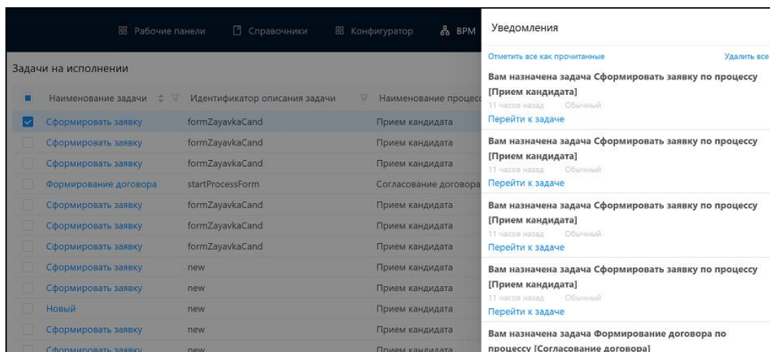
Рисунок 10.51 – Лента уведомлений
