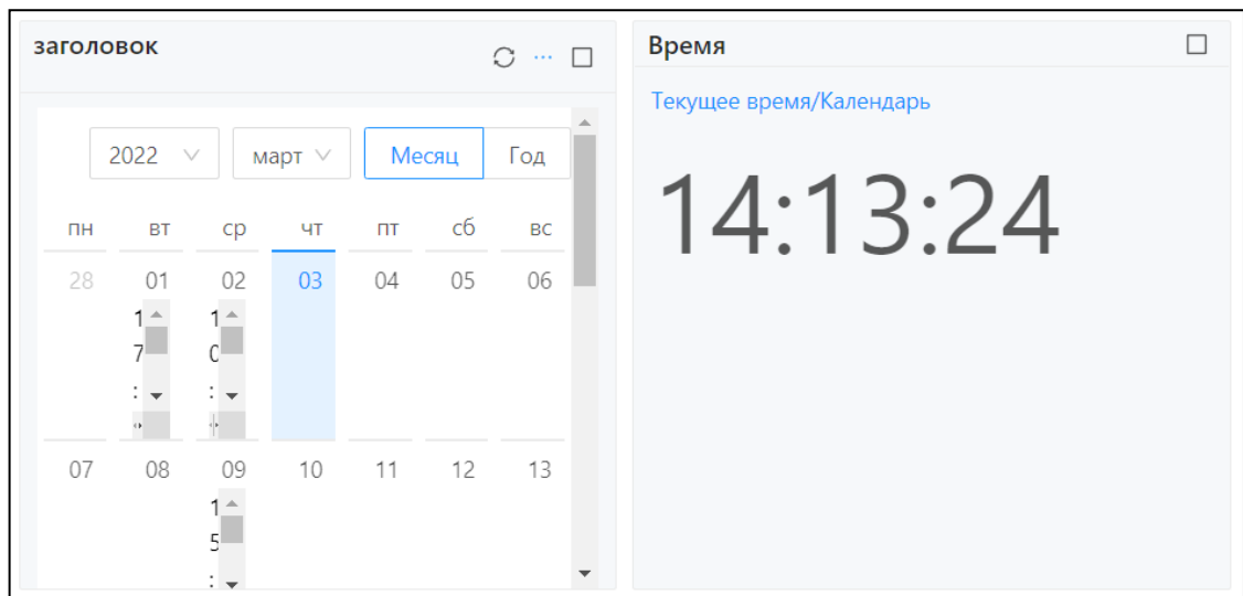
Рисунок 13.5 – Предпросмотр панели
