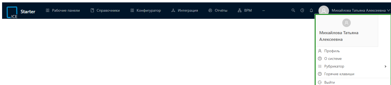
Рисунок 2.45 – Меню пользователя
