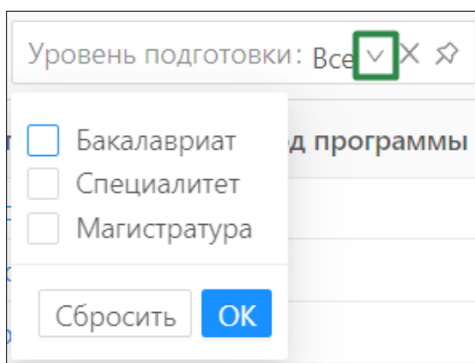
Рисунок 4.54 – Изменение фильтра
