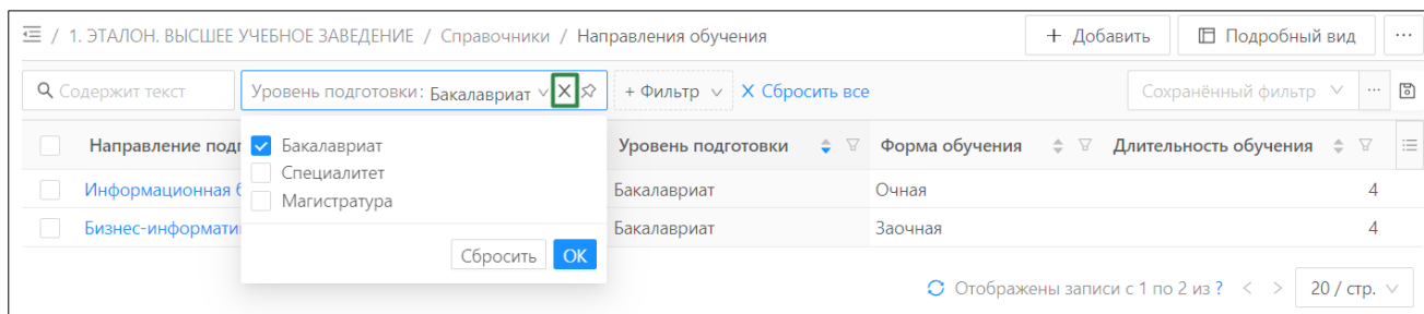
Рисунок 4.53 – Сброс фильтрации
