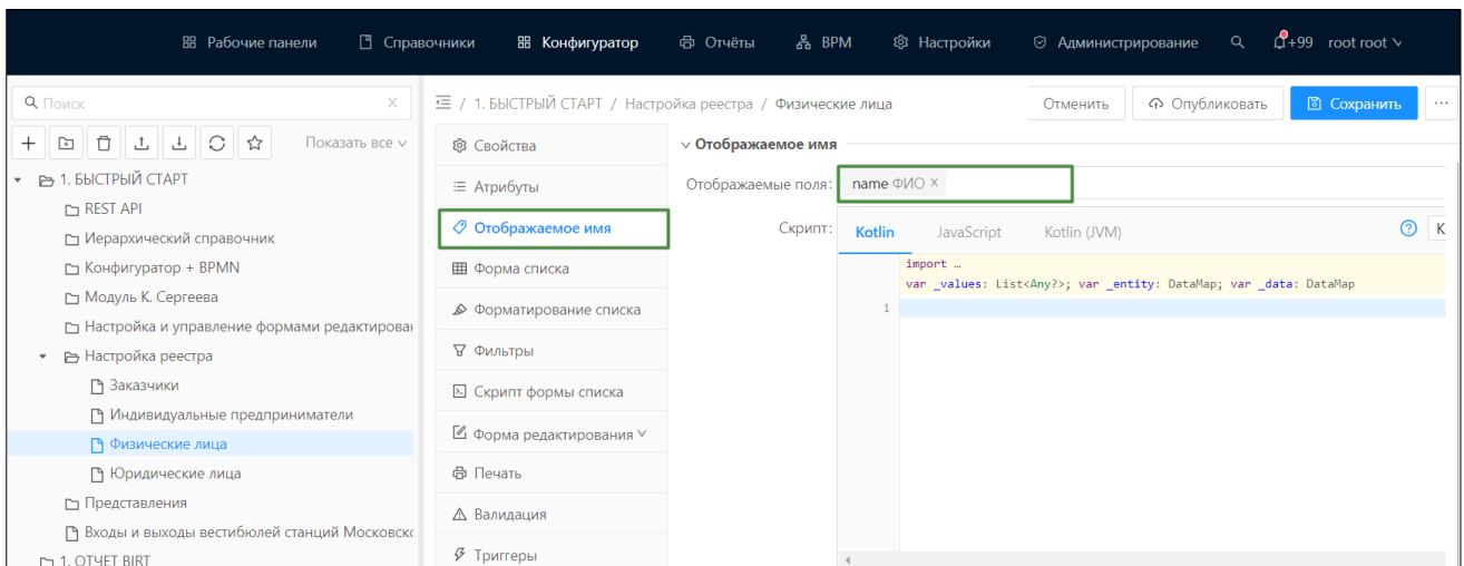
Рисунок 6.13 – Настройка конфигурации объекта приложения на вкладке «Отображаемое имя»
