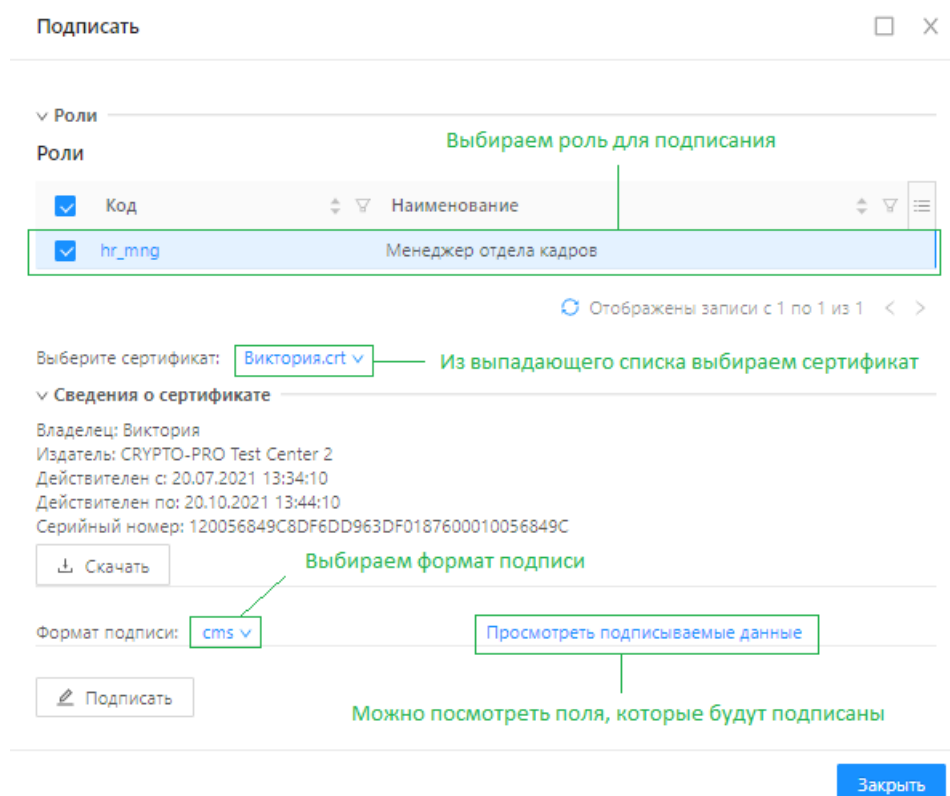
Рисунок 6.102. Форма для подписания экземпляра объекта приложения
