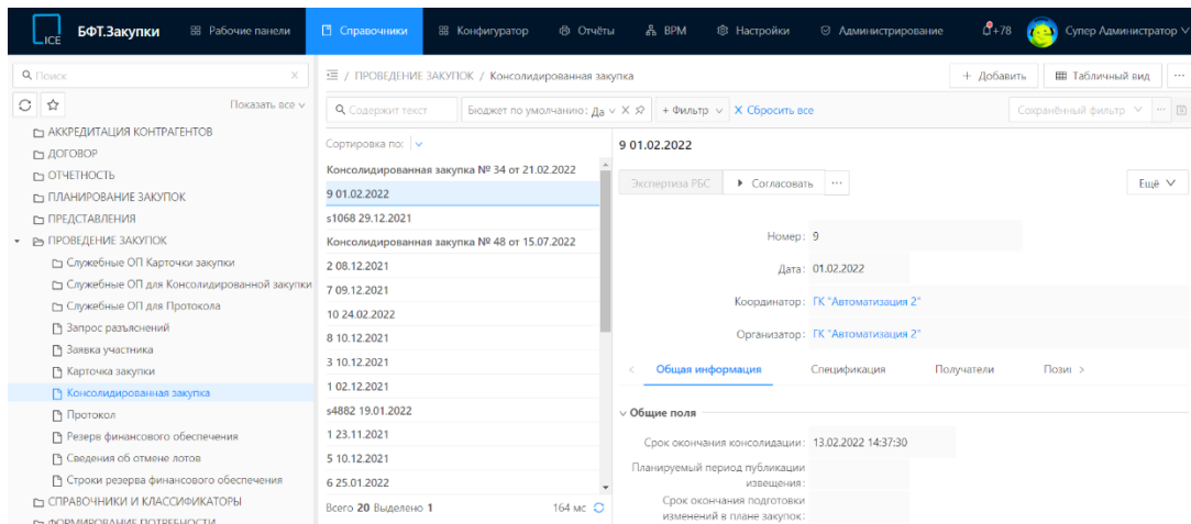
Рисунок 4.37. Форма списка справочника в виде AG Grid в подробном режиме просмотра
