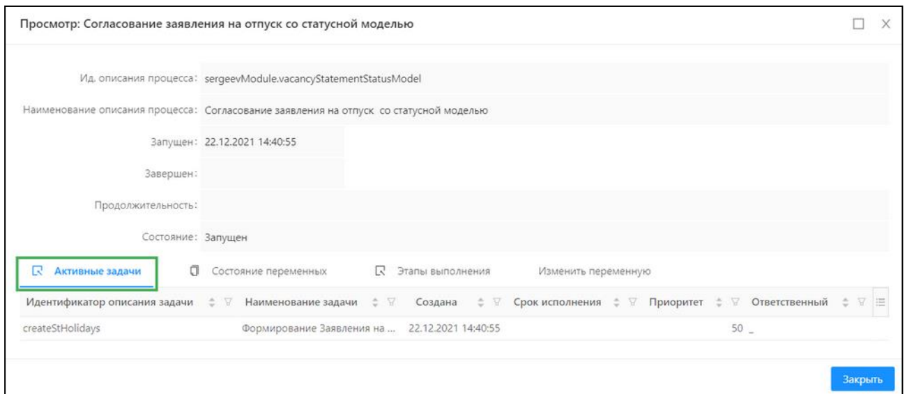
Рисунок 9.83 – Вкладка «Активные задачи» экземпляра процесса
