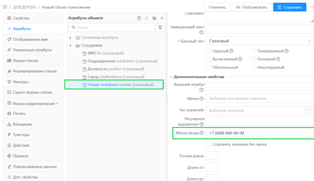
Рисунок 4.40 – Пример заполнения свойства маски ввода для атрибута
