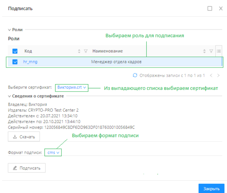
Рисунок 6.110. Форма подписания экземпляра объекта приложения
