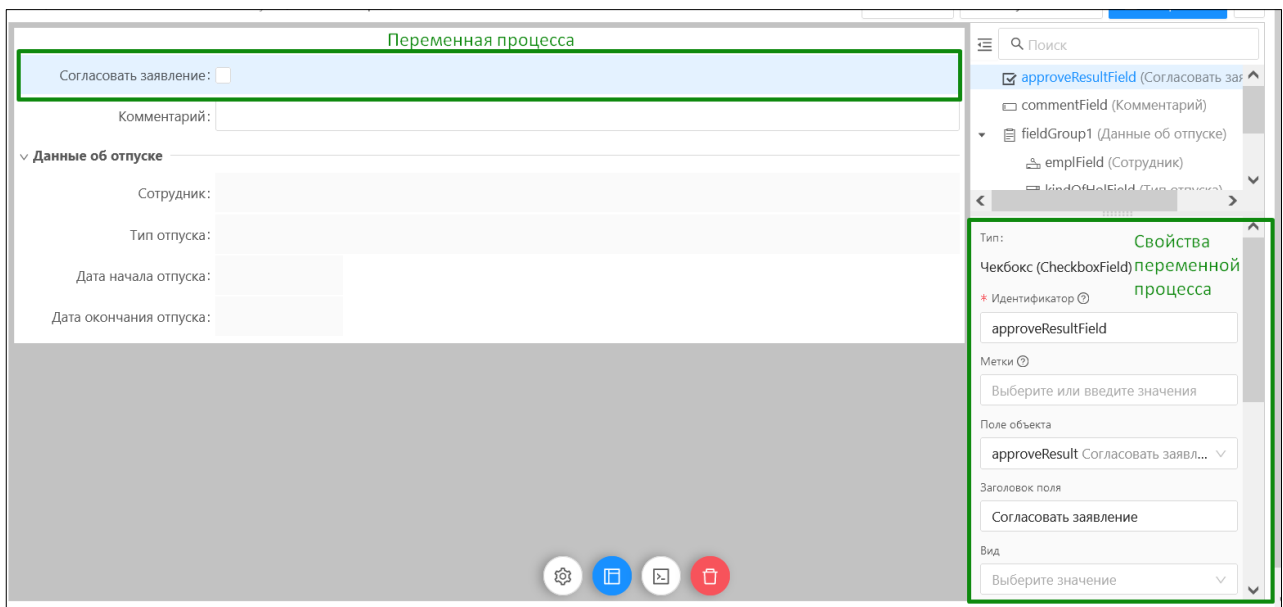
Рисунок 9.26 – Свойства переменных процесса на форме редактирования контекстного объекта приложения
