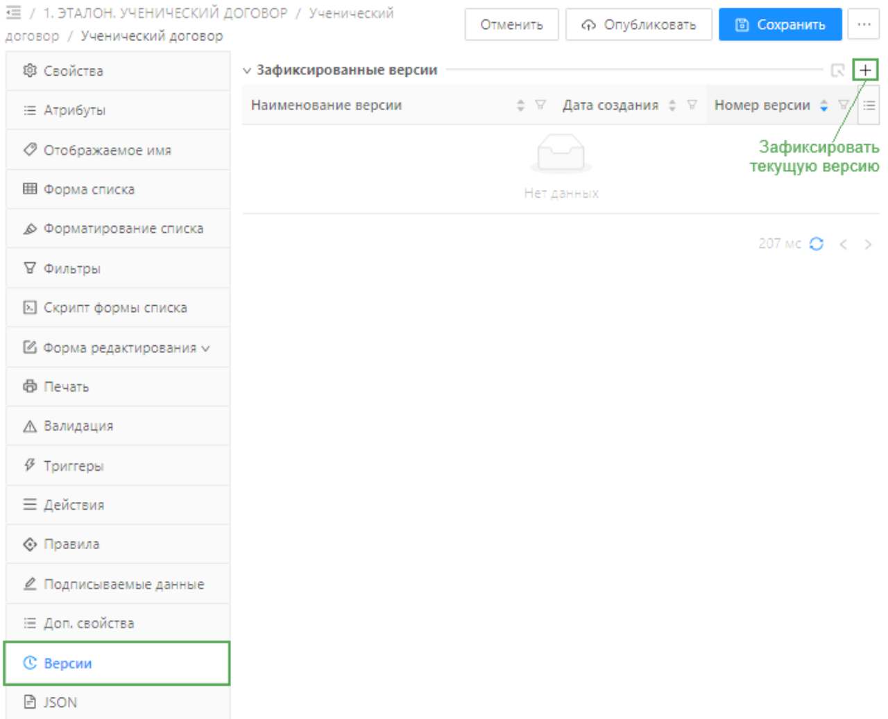
Рисунок 6.79 - Форма редактирования конфигуратора вкладка «Версии»
